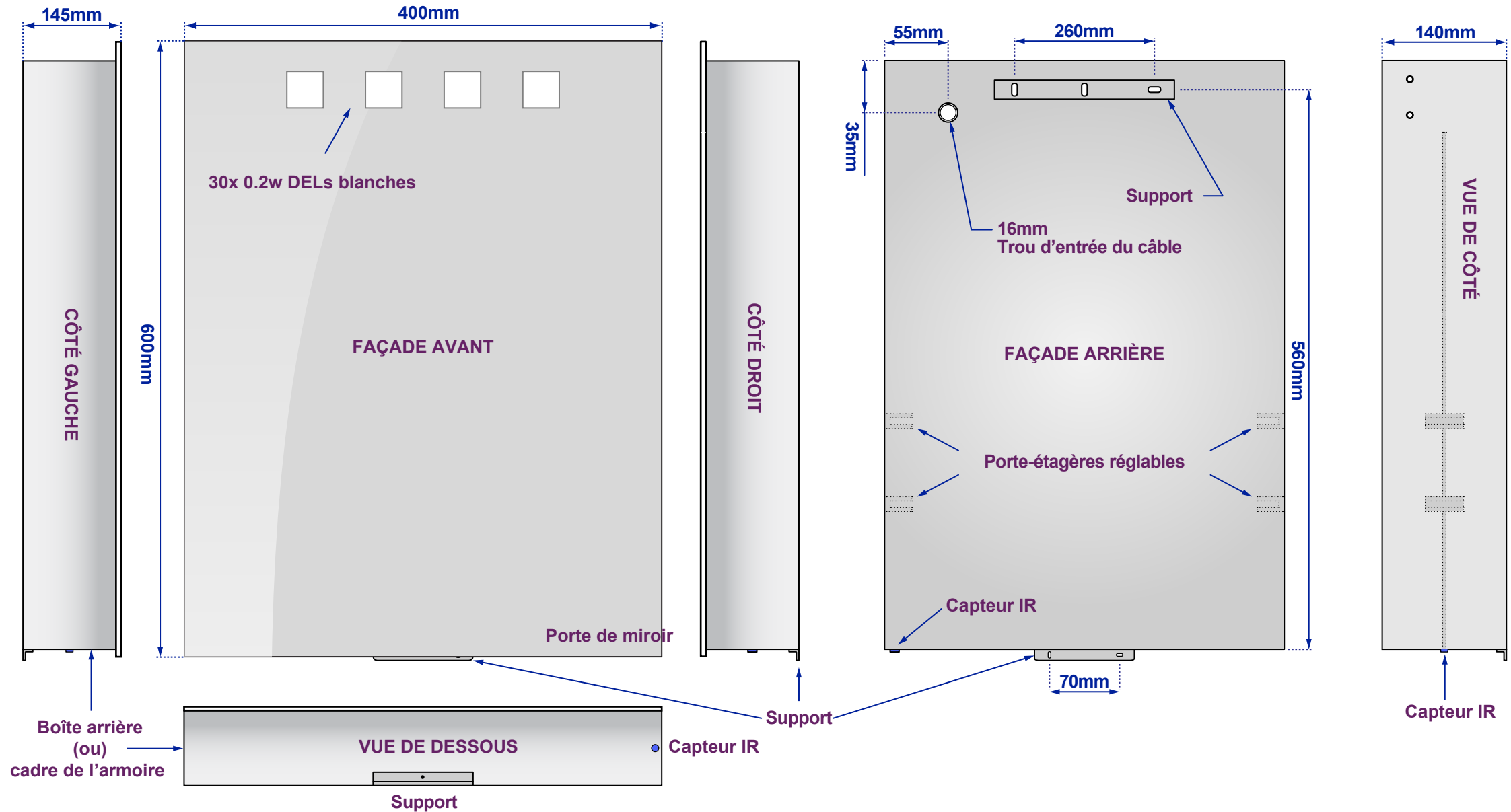
Vues avant et arrière de la boîte arrière – Sans porte-miroir
